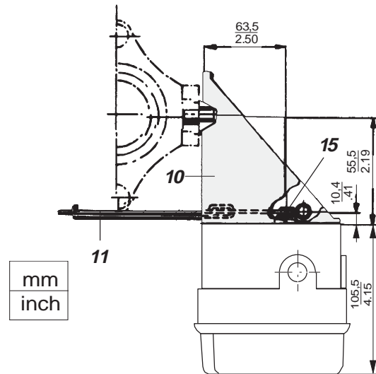
Fig. 10: Montaje en accionamientos de membrana con linterna de fundición según DIN IEC 534-6 (montaje a la derecha), código G
