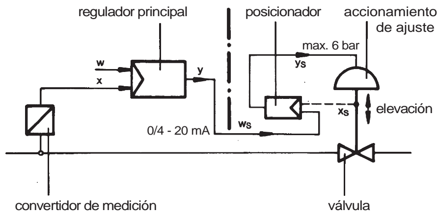
Fig. 1: Circuito regulador con posicionador de acción simple
