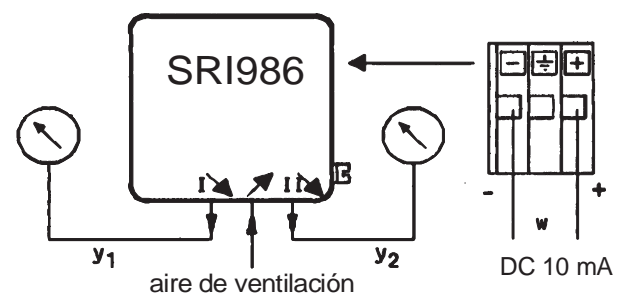
Fig. 25: Circuito de prueba
