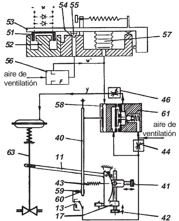
Fig. 2: Posicionador electro neumático de acción simple
