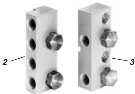
Fig. 5: Regletas de contacto
