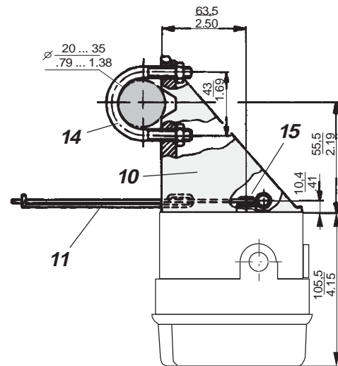
Fig. 11: Montaje en accionamientos de membrana con linterna de pilar según DIN IEC 534-6 (montaje a la derecha), código F
