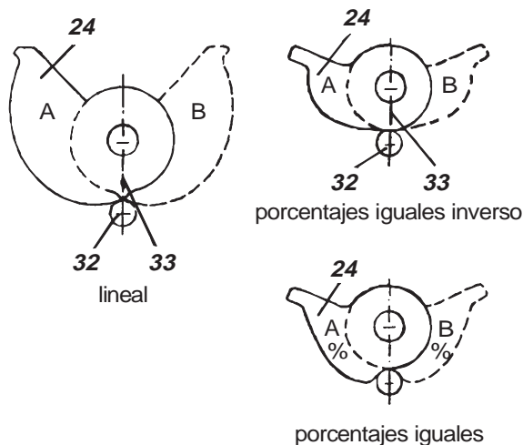
Fig. 18: Alineación de los discos dentados 24
