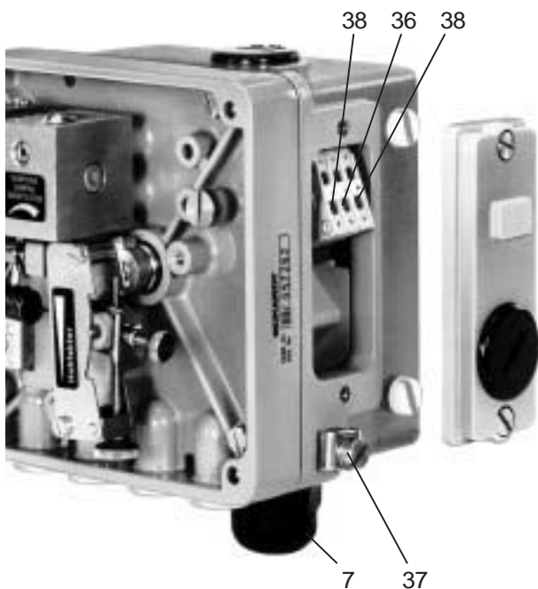
Fig. 21: Conexiones eléctricas
